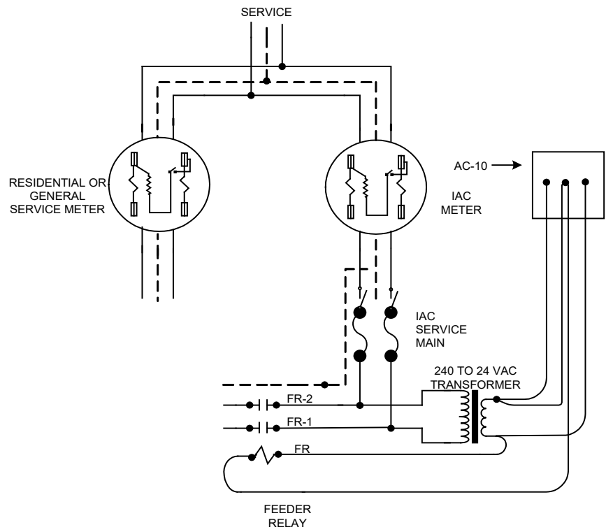
WIRING SCHEMATIC
